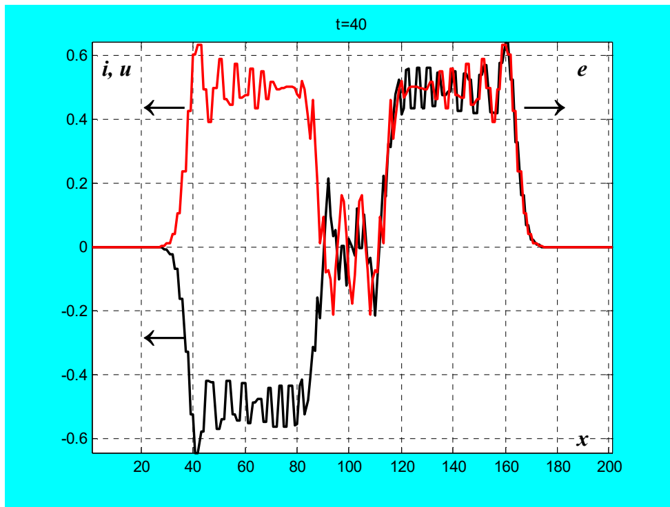
Рис. 2.11. Идеальная линия: R = G = 0 при 0 < x < 200 . Распределение потенциала u (кривые красного цвета) и тока i (черный цвет) в линии на моменты времени: t = 20; 40 .
